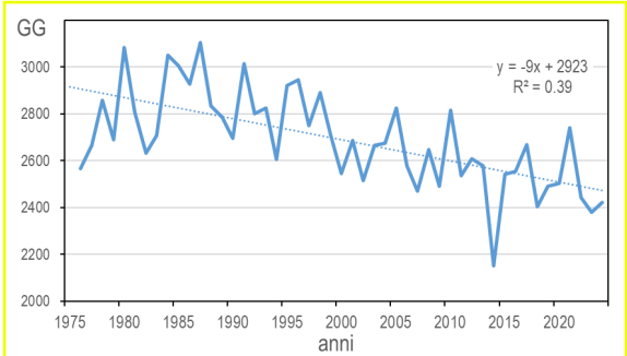
Fig. 1 – Udine: Gradi giorno di riscaldamento (HDD) nell'intero anno solare per gli anni 1976- 2024
