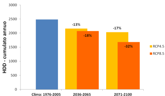
Figura 2 – Gradi giorno di riscaldamento (HDD) nel trentennio 1976-2005, e proiezioni degli stessi sui trentenni 2036-2075 e 2071-2100, scenari emissivi RCP4.5 e RCP 8.5, per Bologna.
