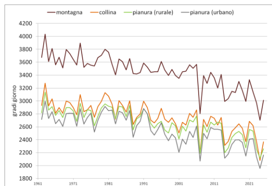
Figura 1 – Gradi giorno di riscaldamento (HDD) nel periodo 1961-2025 nel territorio dell'Emilia-Romagna, suddiviso in aree omogenee.
