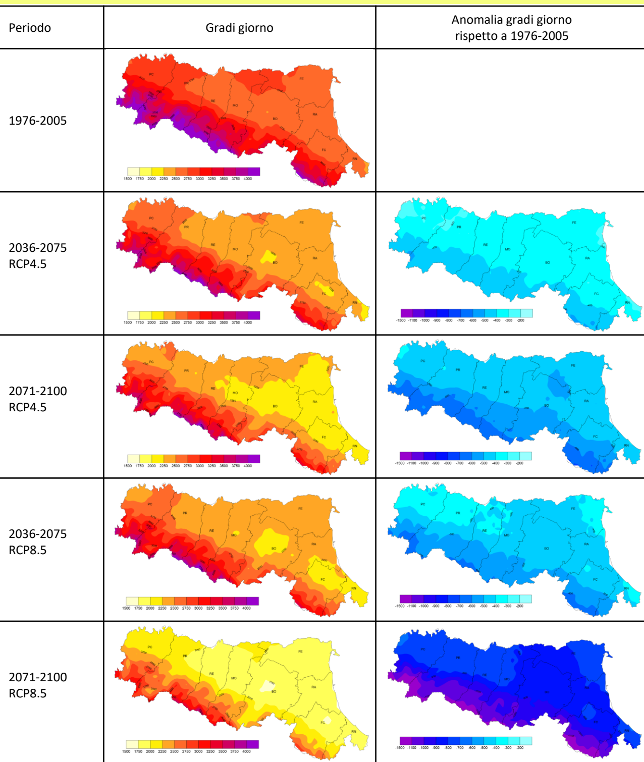
Figura 3 – Gradi giorno di riscaldamento (HDD) nel trentennio 1976-2005, e proiezioni degli stessi sui trentenni 2036-2075 e 2071-2100 per gli scenari di emissione RCP4.5 e RCP8.5, e relative anomalie.
