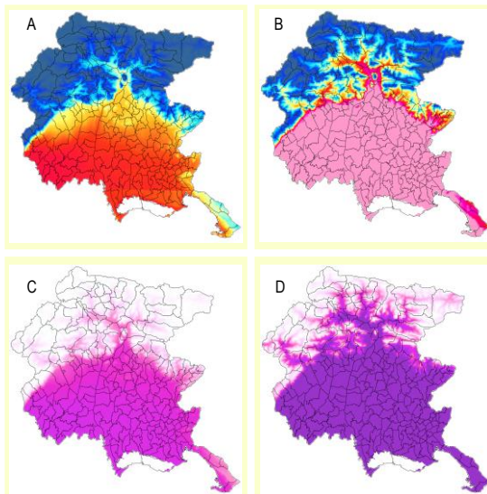
Fig. 5 – Andamenti territoriali medi di CDD (sopra A-B) e anomalia versus 1976-2005 (sotto C-D) nei periodi 2036-2065 e 2071-2100 da proiezioni climatiche nello scenario emissivo RCP8.5
