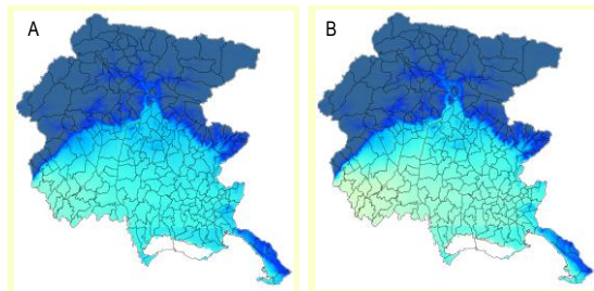
Fig. 3 – Andamenti territoriali medi di CDD nei due trentenni storici 1976-2005 (A) e 1991-2020 (B)
