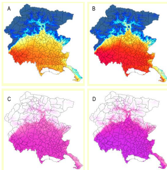
Fig. 4 – Andamenti territoriali medi di CDD (sopra A-B) e anomalia versus 1976-2005 (sotto C-D) nei periodi 2036-2065 e 2071-2100 da proiezioni climatiche nello scenario emissivo RCP 4.5
