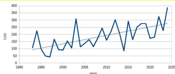
Figura 1 – Legnaro (PD): Gradi giorno di raffrescamento (CDD) nell'anno solare per gli anni 1993-2024.
