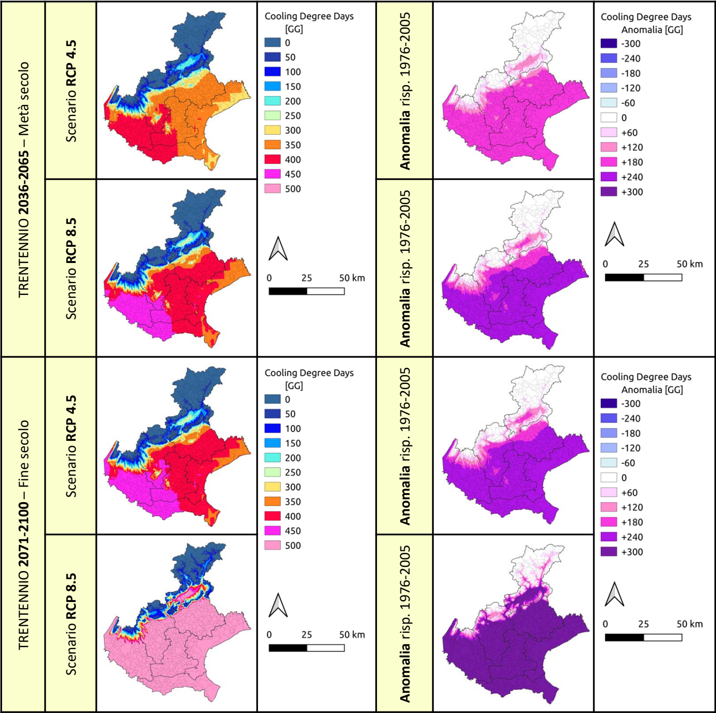
FIG. 4 MAPPE DI PROIEZIONI CLIMATICHE E ANOMALIA
