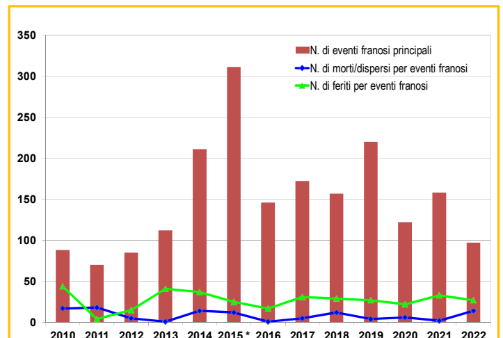
Figura 2 – N. di eventi franosi principali, n. di morti/dispersi e n. di feriti per eventi franosi dal 2010 al 2022.
