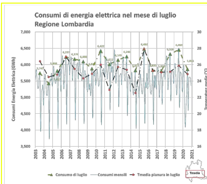
Figura 1 - Consumo mensile di energia elettrica in Lombardia, anni 2003-2020. In linea tratteggiata, il consumo e le temperature medie in pianura del mese di luglio.
